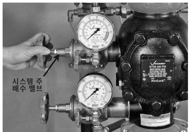
8. 시스템 주 배수 밸브를 열어, 고여있는 물을 배출하고 시스템 에어 압력을 릴리스하십시오.
