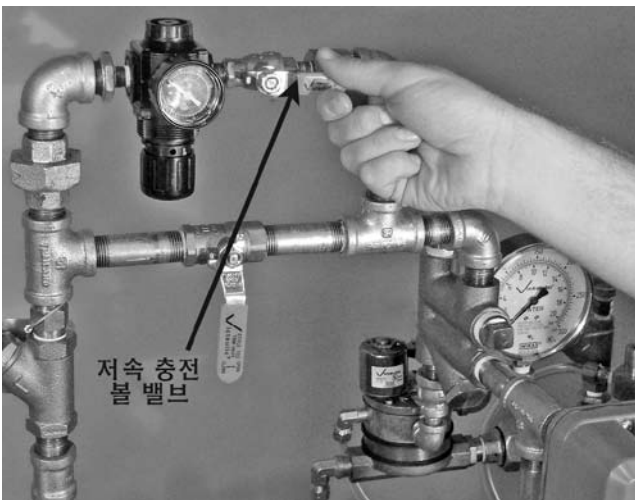
12. Series 757 에어 공급트림 어셈블리(에어 레귤레이터 부착형)의 저속 충전 불 밸브를 여십시오.
