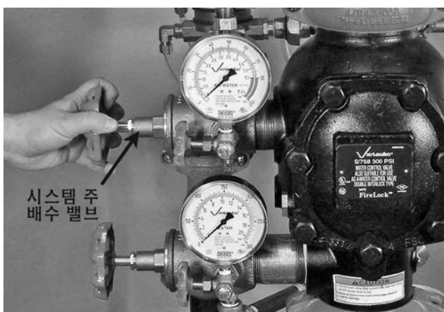
6. 시스템 주 배수 밸브를 일부분만 천천히 여십시오. 배수구에서 물이 흐르지 않는지 확인하십시오. 참고: 배수구에서 물이 흐를 경우, 시스템의 배수준비가 제대로 되지 않을 경우일 수 있으니 "시스템 작동" 섹션에 나오는 단계들을 이행하십시오.
