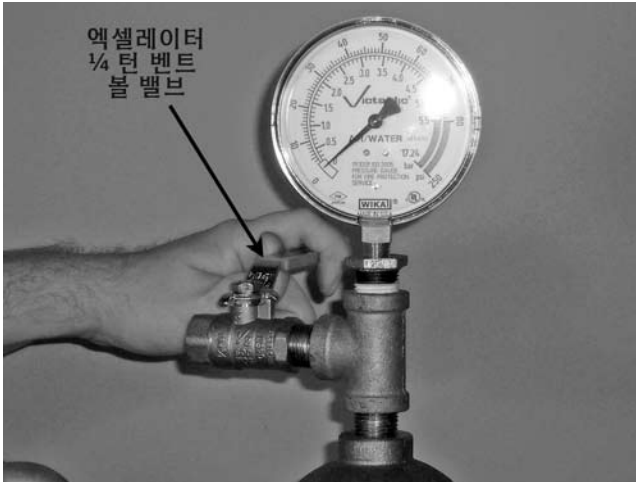
20. Series 746-LPA 드라이 액셀레이터가 설치되면, 1/4-턴 볼 밸브를 닫으십시오.
