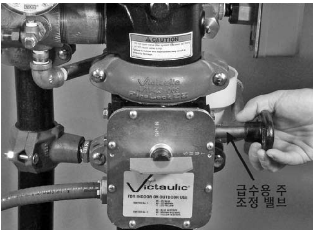
27. 물이 드립 체크로부터 흘러나오면, 급수용 주 조정 밸브를 닫고 1단계에서 다시 시작하십시오. "문제해결" 섹션을 참조하십시오.
