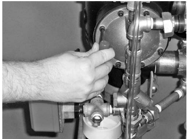
6. 다이어프램을 Victaulic이 공급한 새 다이어프램으로 교체하십시오. 다이어프램의 구멍과 밸브 본체의 구멍을 잘 맞추십시오. 설치 도중 다이어프램에 손상이 가지 않도록 주의하십시오.
