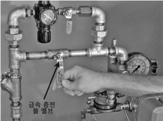
11. 정상 수준의 시스템 에어 압력에 이르면, Series 757 에어 공급트림 어셈블리(에어 레귤레이터 부착형)의 급속 충전 불 밸브를 닫으십시오.
