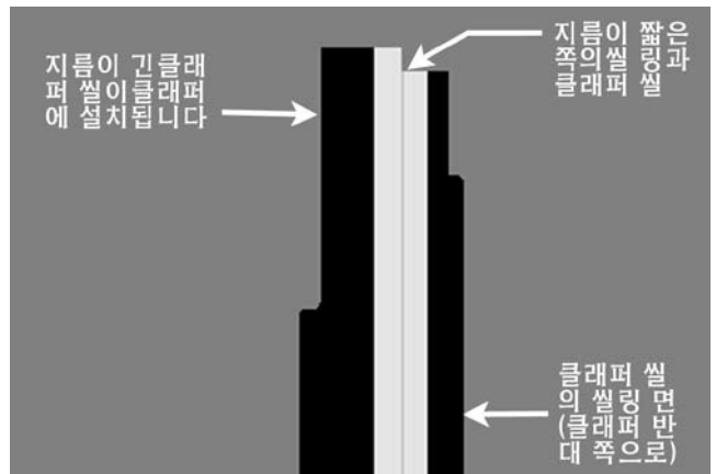
6a. 같은 클래퍼 씰 어셈블리를 이용하여, 이전 단계에서 씰 링이 클래퍼 씰에서 빼내어졌을 경우: 씰 링을 조심스럽게 클래퍼 씰의 바깥쪽 날 밑에 다시 넣으십시오. 지름이 짧은 쪽의 씰링이 클래퍼 씰을 봉인한 표면을 향하고 있는지 확인하십시오.
