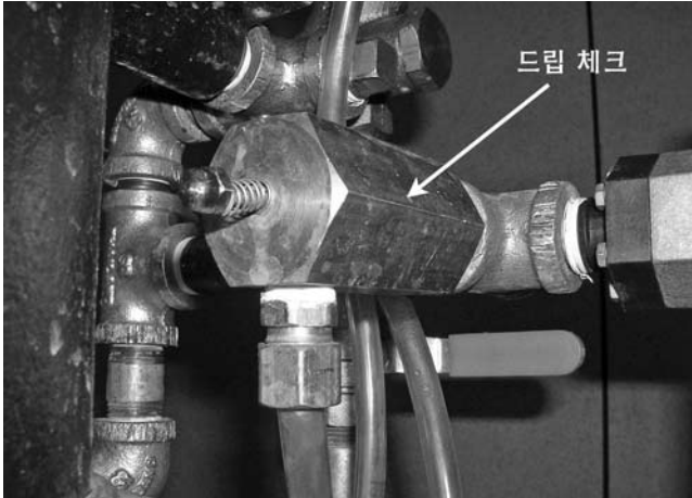
26. 중간 밸브 챔버에서 새는 곳이 없는지 확인하십시오. 알람 라인의 드립 체크는 물 또는 에어를 누출해서는 안 됩니다.
