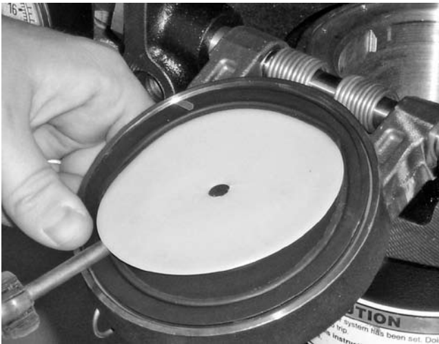
6a. 같은 클래퍼 씰 어셈블리를 이용하여, 이전 단계에서 씰 링이 클래퍼 씰에서 빼내어졌을 경우: 씰 링을 조심스럽게 클래퍼 씰의 바깥쪽 날 밑에 다시 넣으십시오. 지름이 짧은 쪽의 씰링이 클래퍼 씰을 봉인한 표면을 향하고 있는지 확인하십시오.
