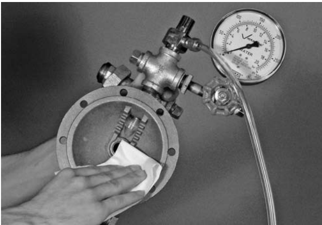
5a. 다이어프램 뒷개 안쪽을 깨끗이 하여 이물질을 제거하십시오.
